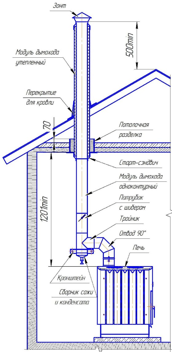
Установка печи
